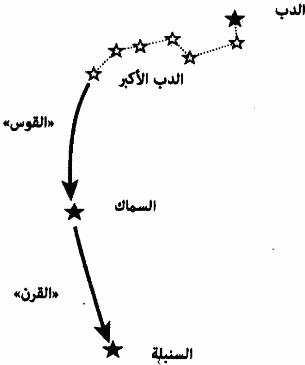
الشكل (49): تحديد النجوم: الدب والسماك والسنبله. تذكر العبارة «القوس إلى السمك، والقرن إلى السنبله» باتباع قبضة الدب الأكبر في قوس يتجه جنوبا.
